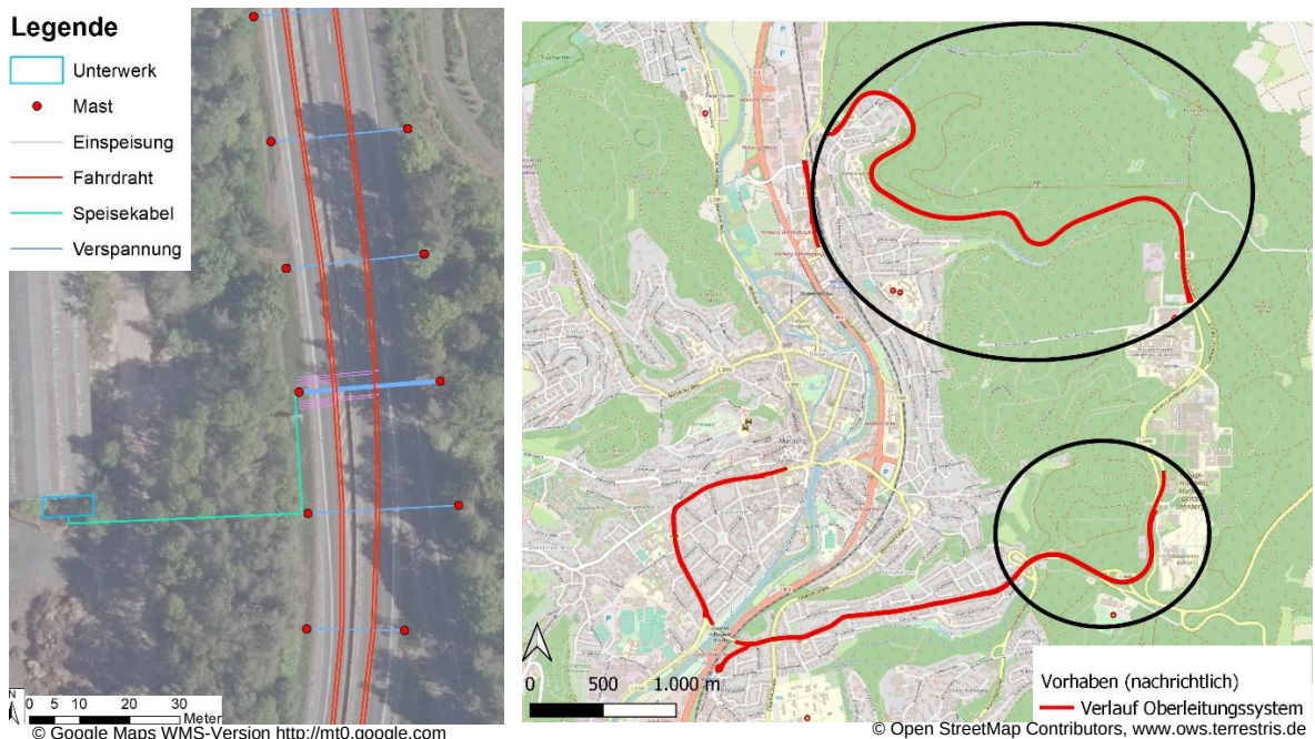
Abbildung 3: Ausschnitt aus der Oberleitungs-Planung (links) sowie Verlauf der Gesamtstrecke (rechts), Quelle: IFB GmbH. Schwarz: Abschnitte der artenschutzrechtlichen Prüfung
